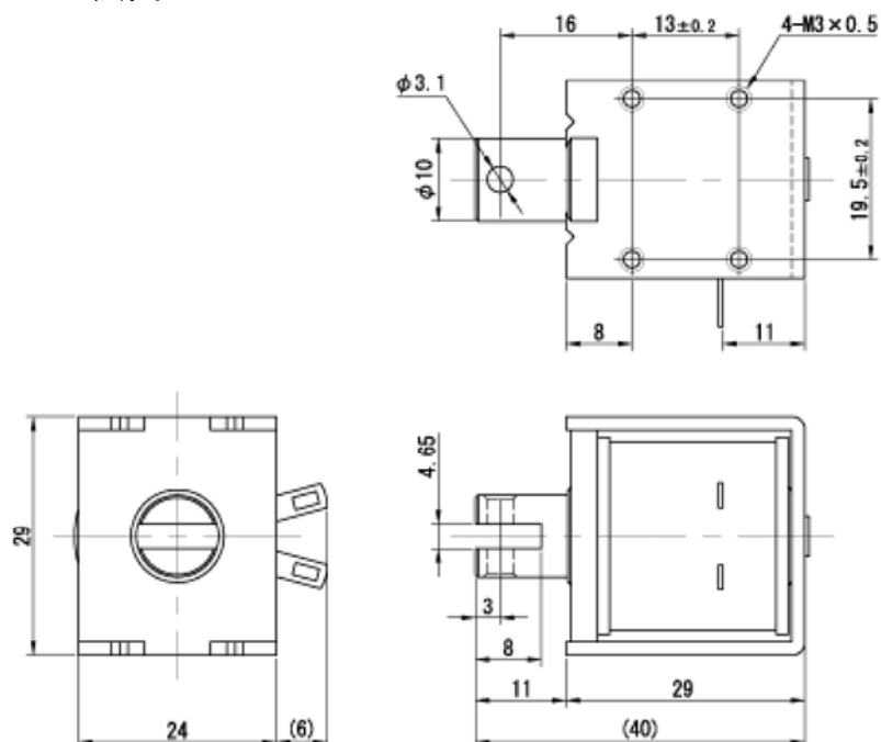
■ 寸法図
