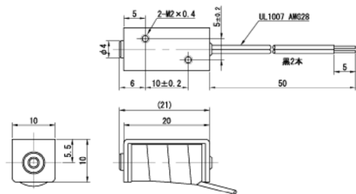
■ 寸法図
